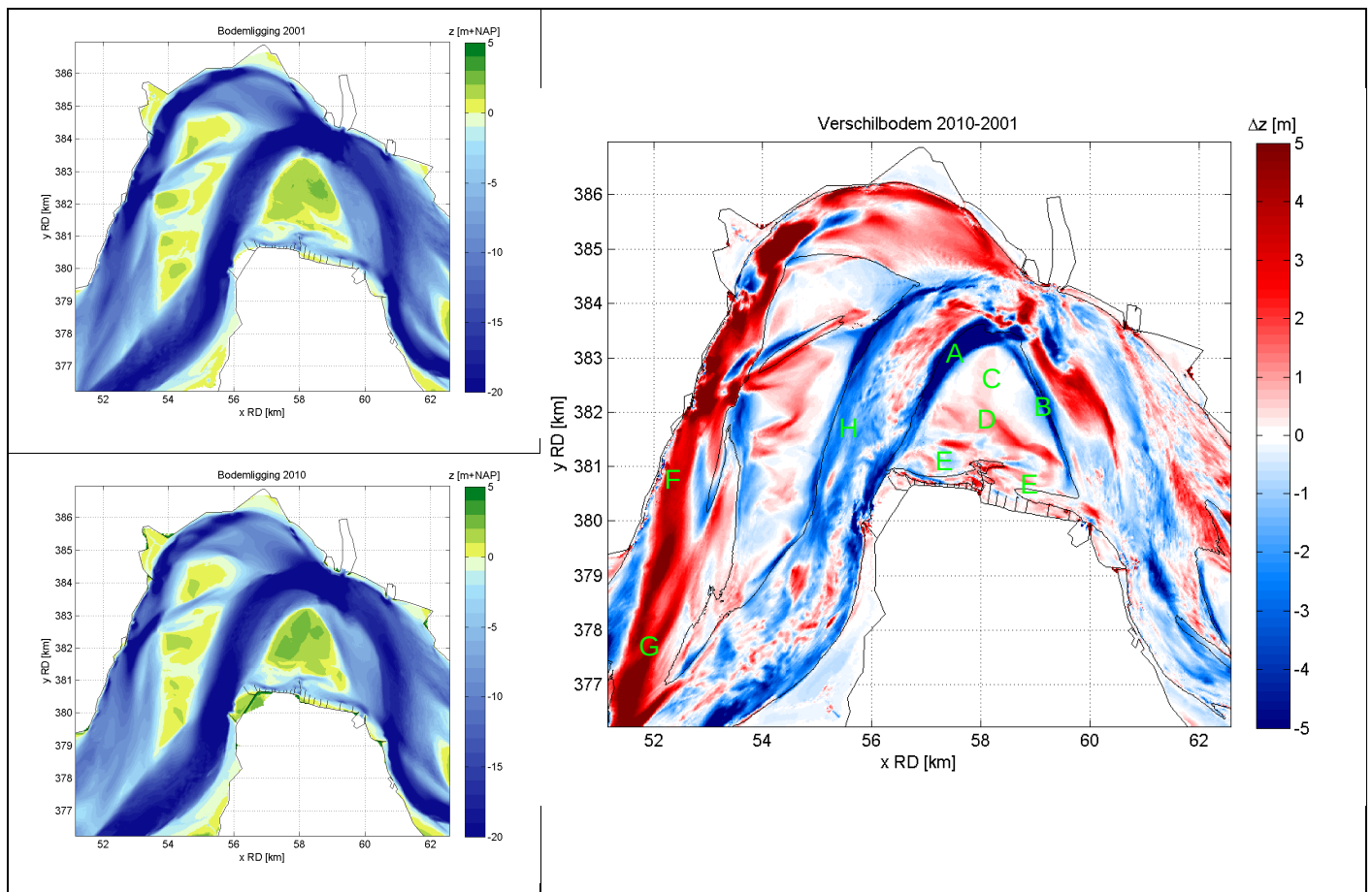
Figuur 2.3 Gemeten bodemligging Platen van Ossenisse in de jaren 2001 en 2010 en verschil in gemeten bodemligging tussen de jaren 2010-2001
