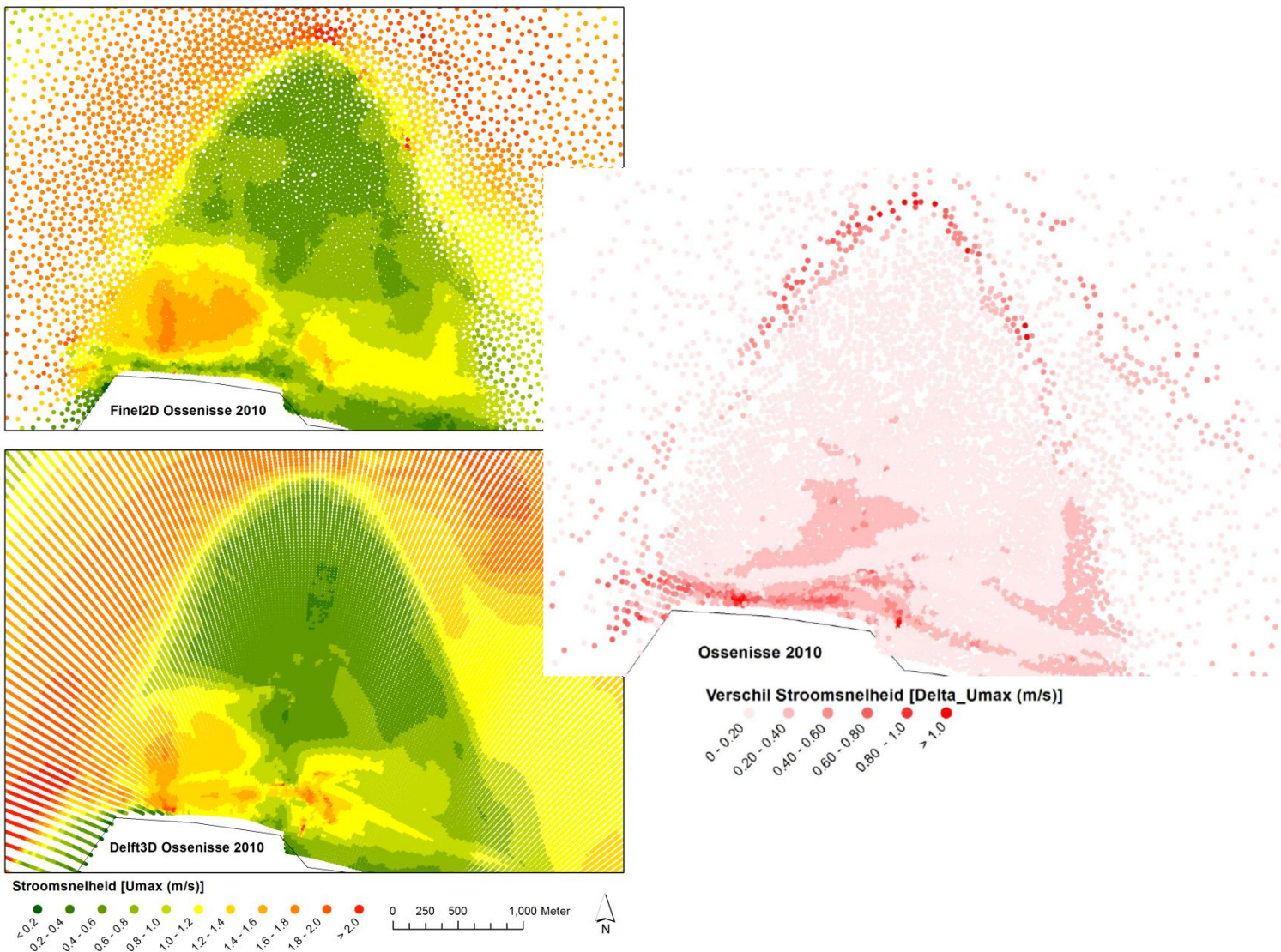
Figuur 3.9 Maximale stroomsnelheid (m/s) nabij de Platen van Ossenissee berekend met FINEL2D (boven) en DELFT3D (onder) en Verschil in Umax tussen FINEL2D en DELFT3D (rechts)
