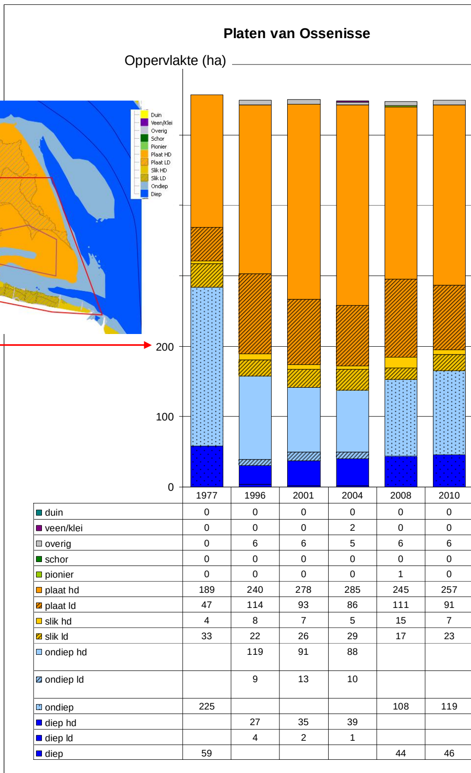
Figuur 2.14 Areaalontwikkeling Ecotopen Platen van Ossensisse
