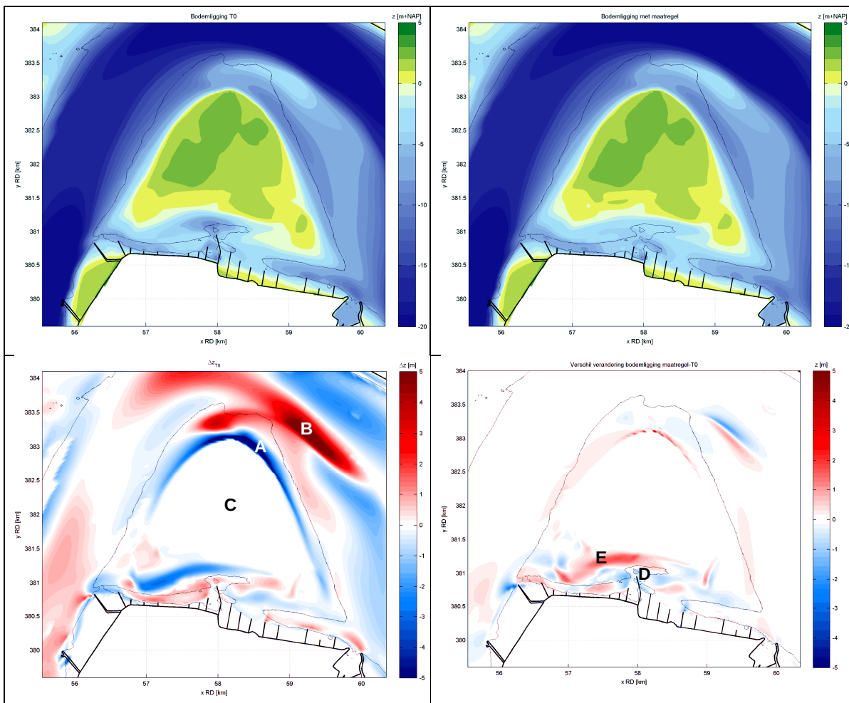
Figuur 4.5 Morfologische situatie na 2 jaar als gevolg van inkorten van de dam berekent met Delft3D. Linksboven: T0-bodemligging. Rechtsboven: bodemligging met ingreep. Linksonder: Verschilbod. zonder ingreep. Rechtsonder: Verschilbod. met ingreep ten opzichte van verschilbod. zonder ingreep.
