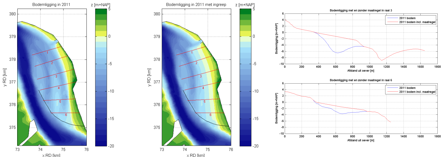
Figuur 4.11 T0 beginsituatie (links) en de beginsituatie van de scenarioberekening (midden) en bodemligging met en zonder maatregel in raaien 3 en 6 (rechts)
