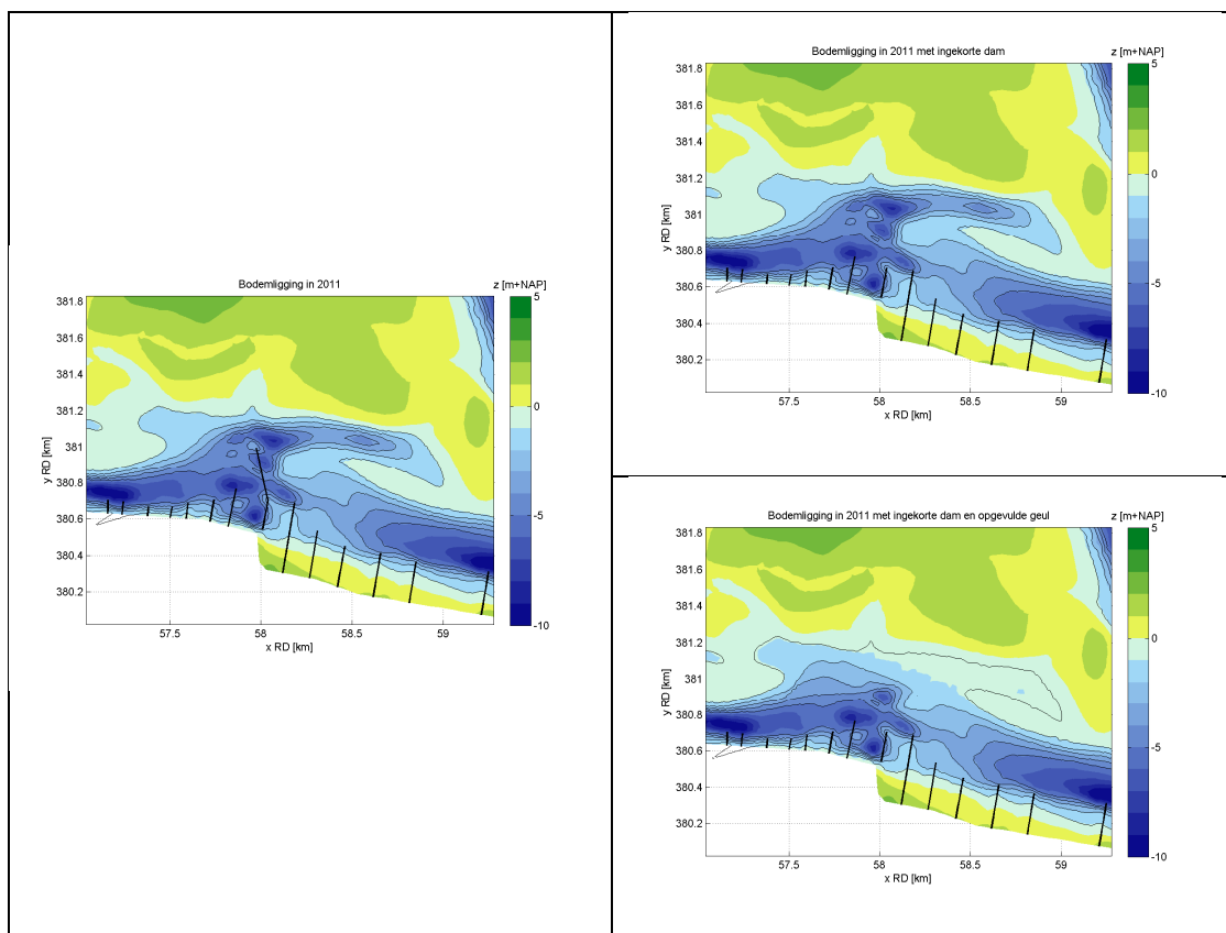
Figuur 4.1 T0 beginsituatie (links), beginsituatie met de ingekorte dam (rechtsboven) en beginsituatie met ingekorte dam en opgevuld geul (rechtsonder)
