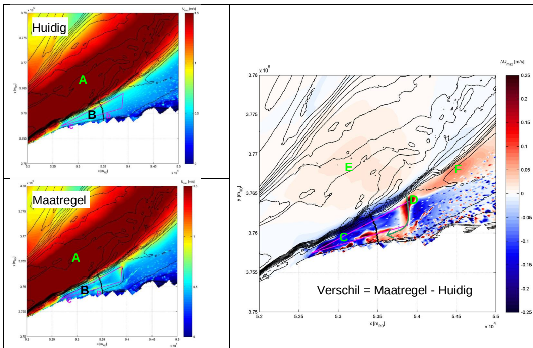
Figuur 4.10 Maximale stroomsnelheid (in m/s) tijdens een springtij-doottij cyclus berekend met Delft3D voor de huidige situatie (2011, linksboven), de situatie na aanleg van 2 m zandlichaam (linksonder) en het verschil tussen beide situaties (rechts, blauw houdt een lagere maximale stroomsnelheid met de maatregel)
