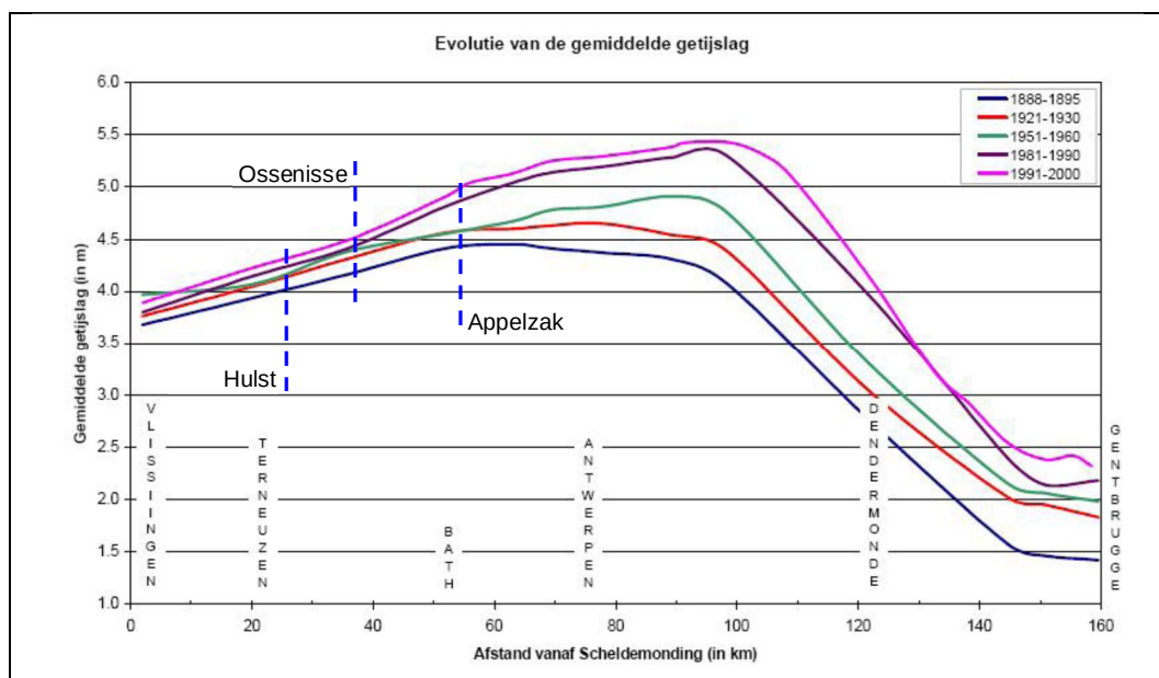
Figuur 2.1 Ontwikkeling getijslag over 120 jaar tot 2000 (Jeuken et al., 2007, op basis van data van Claessens en Meyvis, 1994, en gegevens van E. Taverniers voor de periode 1991-2000).
