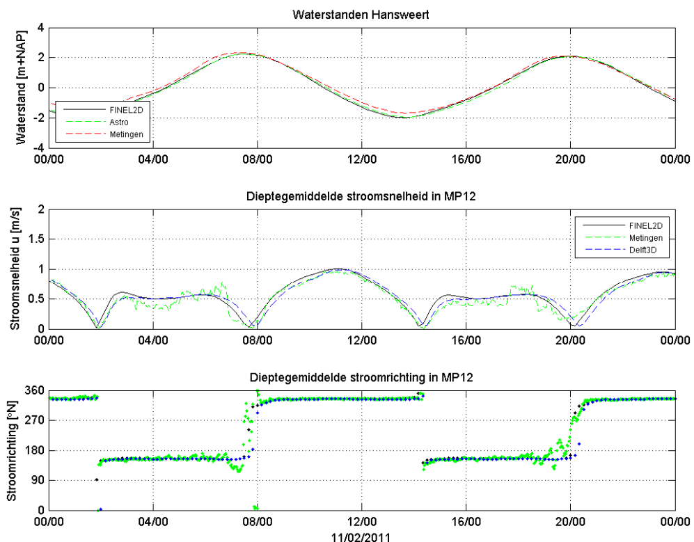
Figuur 3.3 Gemeten met Delt3D en gemodelleerde waterstand (boven) voor locatie Hansweert en stroomsnelheid (midden) en stroomrichting (onder) voor locatie MP12 in het model voor de Platen van Ossenissee.
