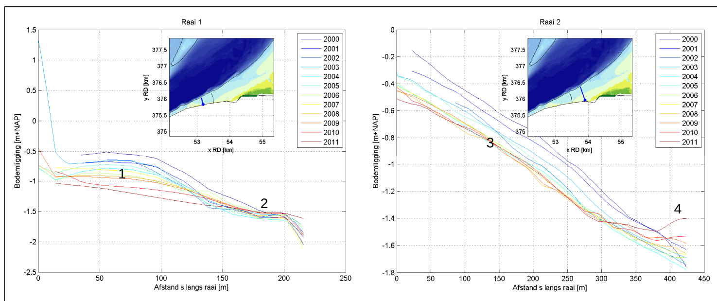
Figuur 2.5 Bodemontwikkeling Slikken van Hulst in twee dwarsraaien. Startpunt van de raai (s=0) is aangegeven met de blauwe punt in de inzet. NB: Schaal x-as en y-as zijn niet gelijk voor de twee raaien.
