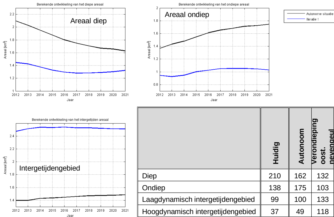
Figuur 4.13 Tijdsree van het diepe (linksboven), ondiepe (rechtsboven) en intergetijden (linksonder) areaal in de periode 2012-2021 voor de autonome situatie en voor de eerste ontwerpiteratie.
