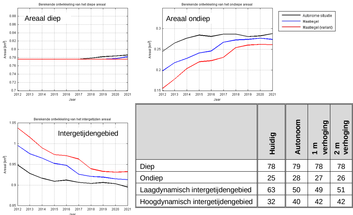
Figuur 4.9 Tijdserie van het diepe (linksboven), ondiepe (rechtsboven) en intergetijden (linksonder) areaal in de periode 2012-2021 voor de autonome situatie, voor de eerste ontwerpiteratie en voor de tweede ontwerpiteratie 2.
