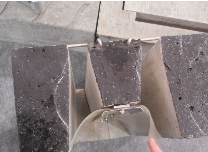
Figuur 30: Inlegroosterbalk voorzien van flappen in dwarsdoorsnede
